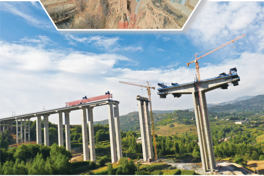
临大高速公路杨家岭大桥位于临夏县营滩乡沙泥锅村和积石山县仇藏镇杨家岭村之间,为左右分离式桥梁,总投资1.8亿元,桥长930米。
